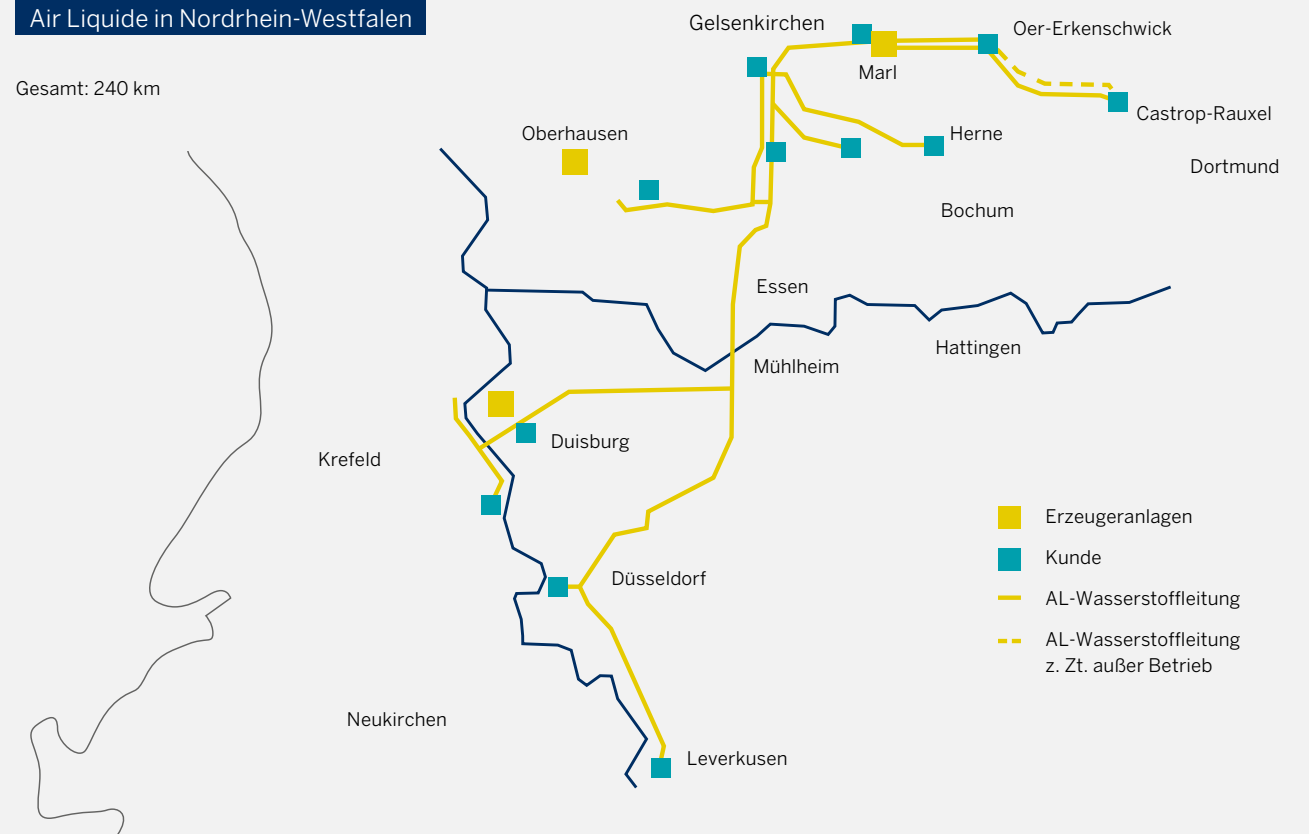
Abbildung 6: Wasserstoffnetz der Air Liquide in Nordrhein-Westfalen
