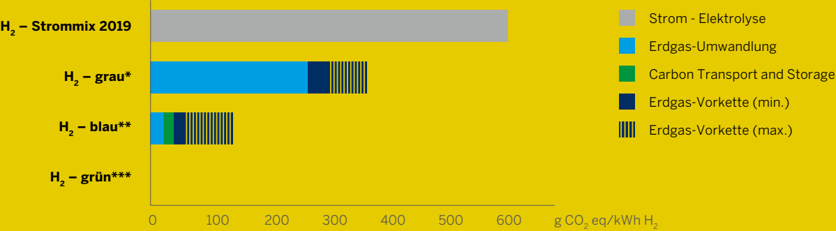
Abbildung 5: CO 2 -Emissionen der verschiedenen Wasserstofffarben
